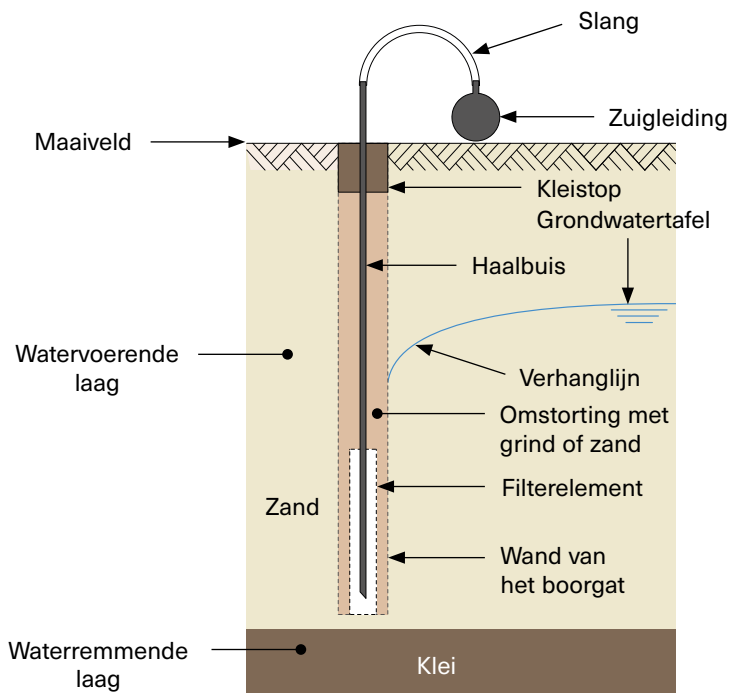
1 Vacuümfilterbemaling van een bouwterrein door verticale filters aangesloten op een zuigerpomp.
